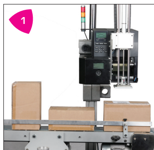
1 Etiquetage sur des objets mobiles de différentes tailles. Jusqu'à 30 étiquettes par minute.
